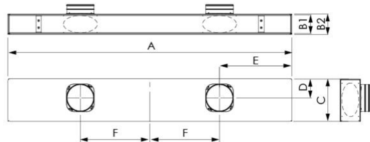
2 INGRESSI / 2 INLET
