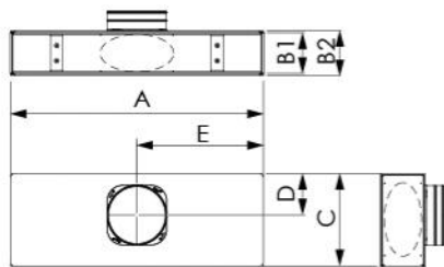
1 INGRESSO / 1 INLET
