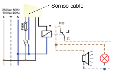
* Il Relè NON è fornito in dotazione. the Relay is NOT supplied
