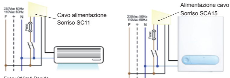
Fuse: 315mA Rapido
