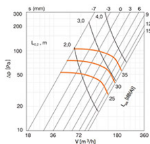
MOD. Ø125
