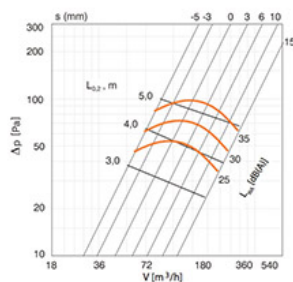
MOD. Ø150
