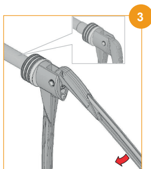
Allargare fino alla battuta (Fig.3) / Press handles together until stop (Pic.3)
