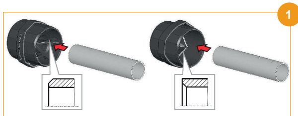
Sbavare il tubo internamente e esternamente (Fig.1) / Debur pipe inside and outside (Pic.1)
