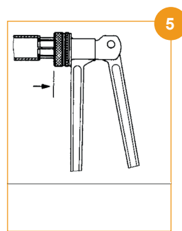
Si possono calibrare tubi deformati nel primo gradino (Fig.5) / Distorted pipe ends can be recalibrated (Pic.5)
