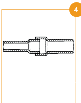
Adatto anche per tubi di diametri diversi (Fig.4) / Also for joining pipes with different diameters (Pic.4)
