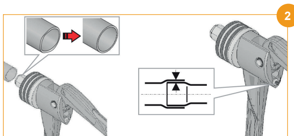
Inserire il tubo fino alla battuta (Fig.2) / Slip on pipe up to the stop (Pic.2)
